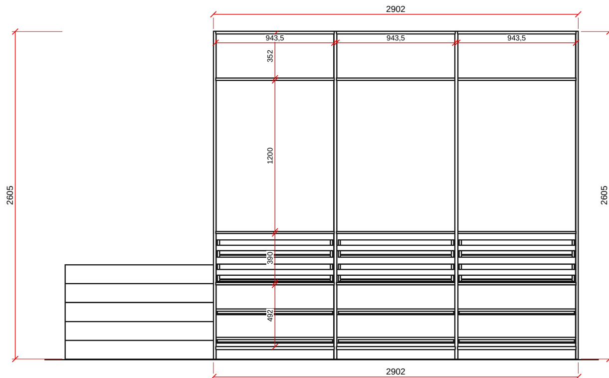
VISTA A - ESC. 1:30
