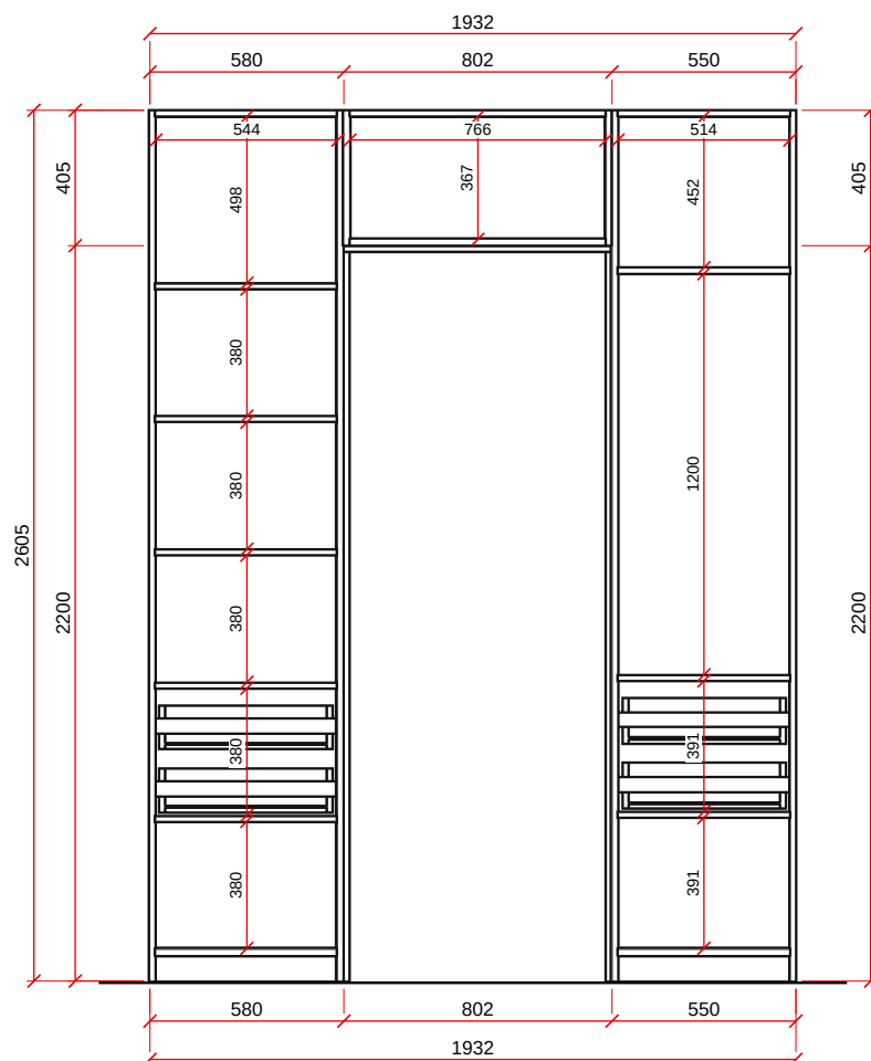
VISTA C - ESC. 1:25
