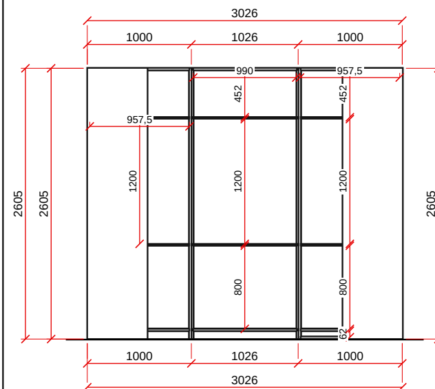
VISTA B - ESC. 1:50
